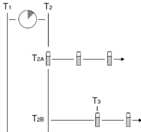
Figure 3-5 Réglages d'activation
