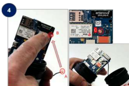
Faire passer le connecteur mâle (A) du fil de l'antenne dans la trou (B) et le connecter à la carte via le connecteur femelle (C)
